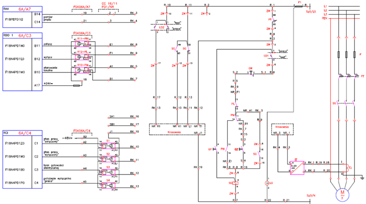
Załącznik nr 2 - Schemat ideowy rozdzielnicy
